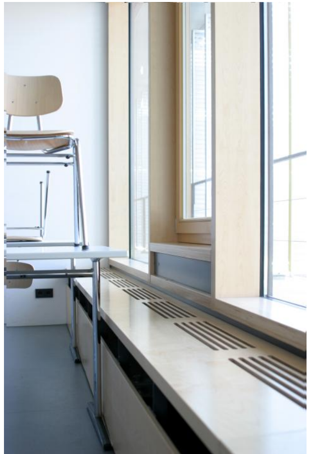
Die Zuluft wird über Brüstungskonvektoren geführt ...
