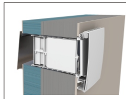
Montagetyp LAW gerade durch die Wand
