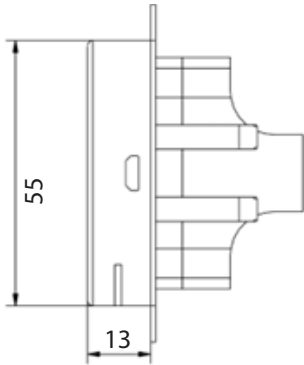
Seitenansicht (rechts)
