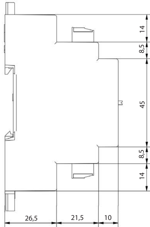
Seitenansicht
