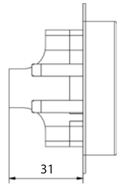
Seitenansicht (links)
