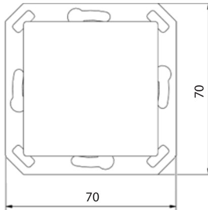
Vorderansicht (raumseitig)
