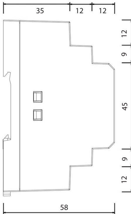
Seitenansicht
