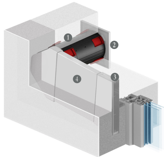
① Wandlüfter bzw. Laibungslüfter ② Innenblende* ③ Fassadenabschluss* ④ Flachkanal (Laibungslüfter)
